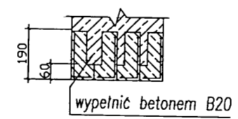
PRZEKROJ A-A 1/20
