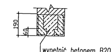
PRZEKROJ B-B 1/20
