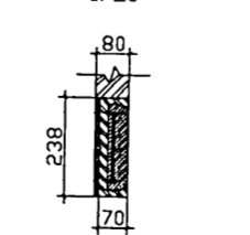
PRZEKROJ C-C 1/20
